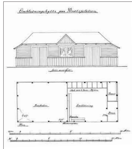
Figur 4. Tegning af omklædningshytten 1916. Nyborg Lokalhistoriske Arkiv.
